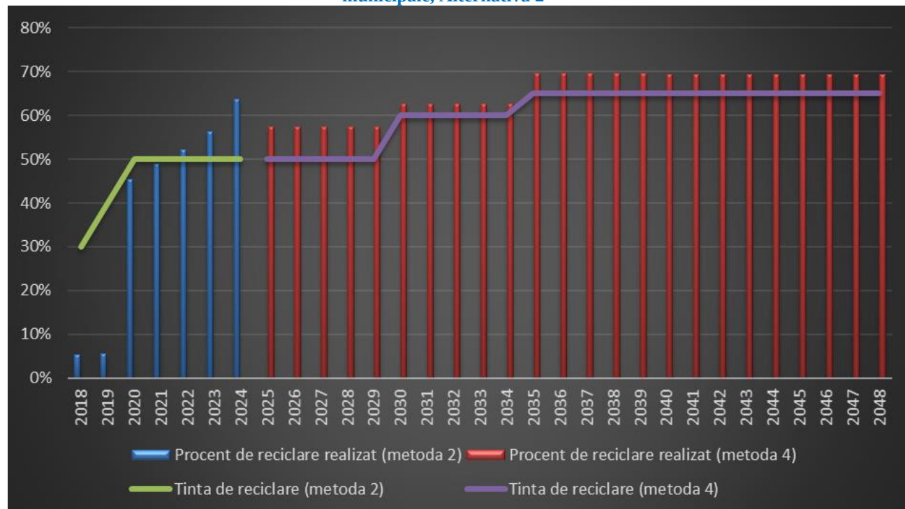
Figura 7-29 Modul de atingere al obiectivului de pregătire pentru reutilizare și reciclare al deșeurilor municipale, Alternativa 2
