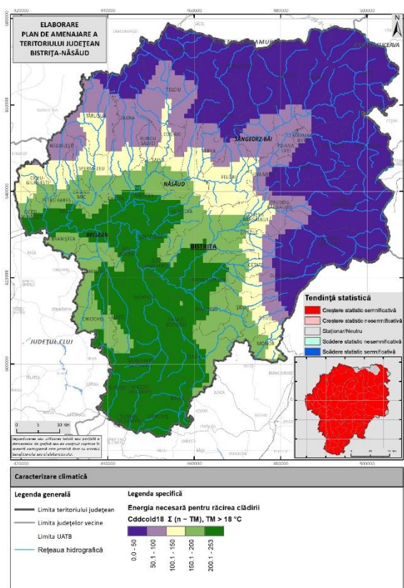
Fig. 2.61. ENERGIA NECESARĂ PENTRU RĂCIREA CLĂDIRILOR (CDDCOLD)
