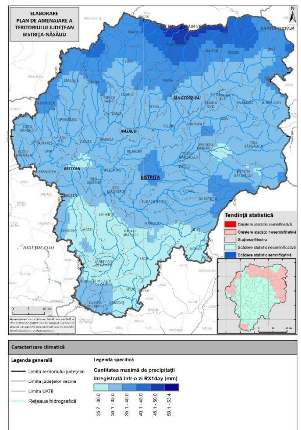
Fig. 2.60. CANTITATEA MAXIMĂ DE PRECIPITAȚII ÎNREGISTRĂ ÎNTR-O ZI
