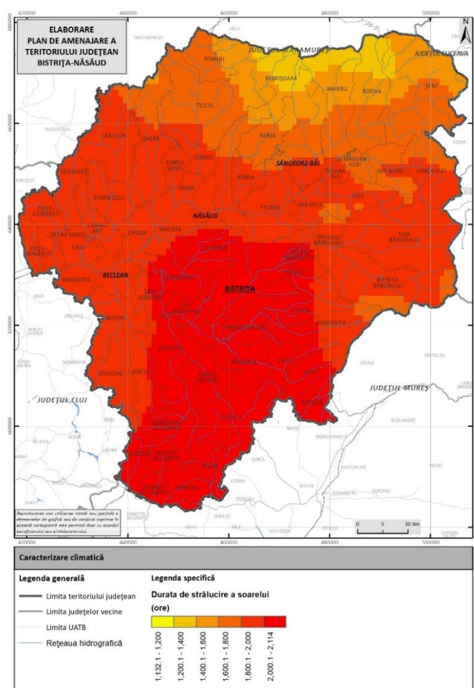
Fig. 2.29. DURATA DE STRĂLUCIRE A SOARELUI ÎN JUDEȚUL BISTRIȚA-NĂSĂUD PENTRU PERIOADA 2004-2024.
