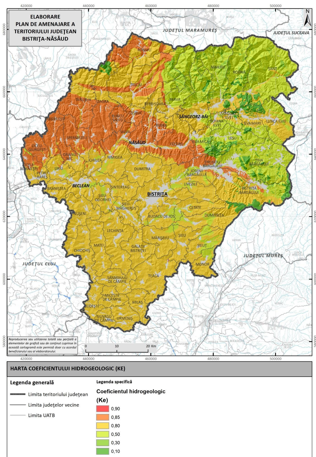
Fig. 2.32. HARTA COEFICIENTULUI HIDROGEOLOGIC (KE)
