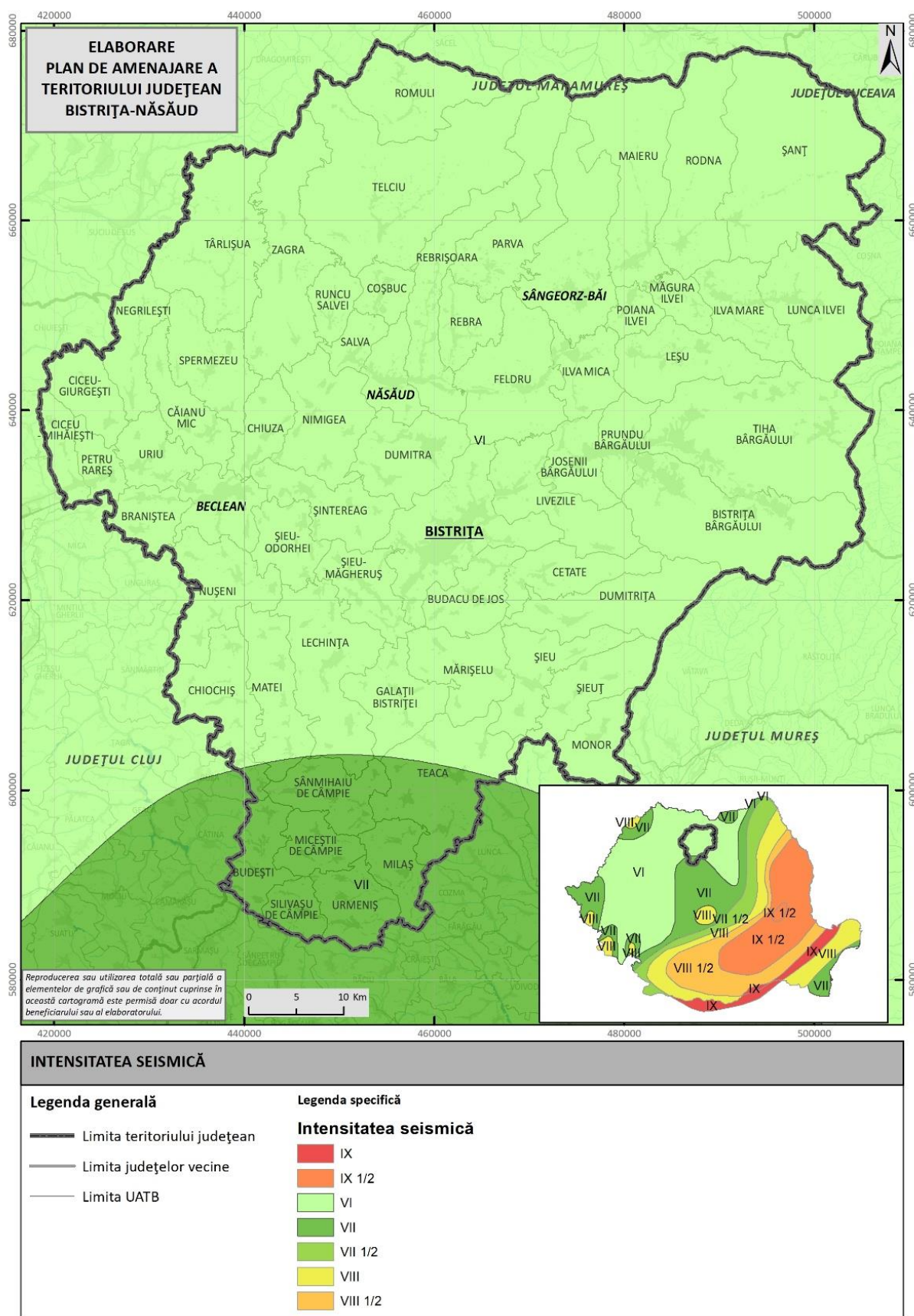
Fig. 2.21. HARTA INTENSITĂȚII SEISMICE (SCARA MSK)
