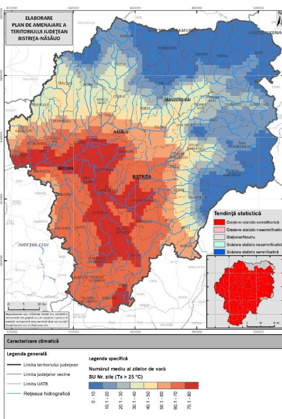
Fig. 2.55. ZILE DE VARĂ
