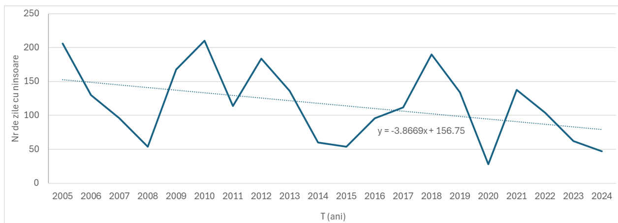
Fig. 2.65. ZILELE CU NINSOARE
