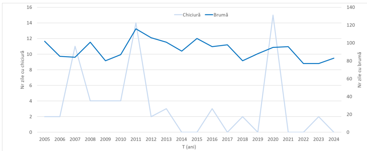
Fig. 2.69. ZILELE CU BRUMĂ ȘI ZILELE CU CHICIURĂ
