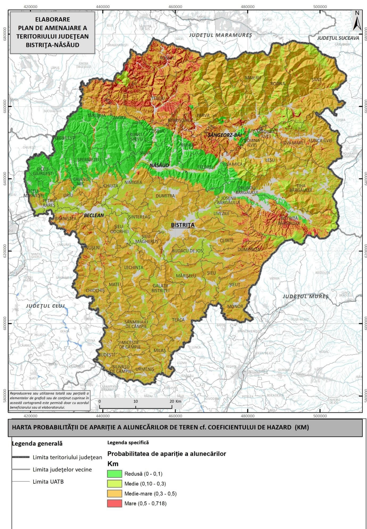
Fig. 2.36. PROBABILITATEA DE PRODUCERE A ALUNECĂRILOR DE TEREN ȘI COEFICIENTUL DE RISC CORESPUNZĂTOR (KM)
