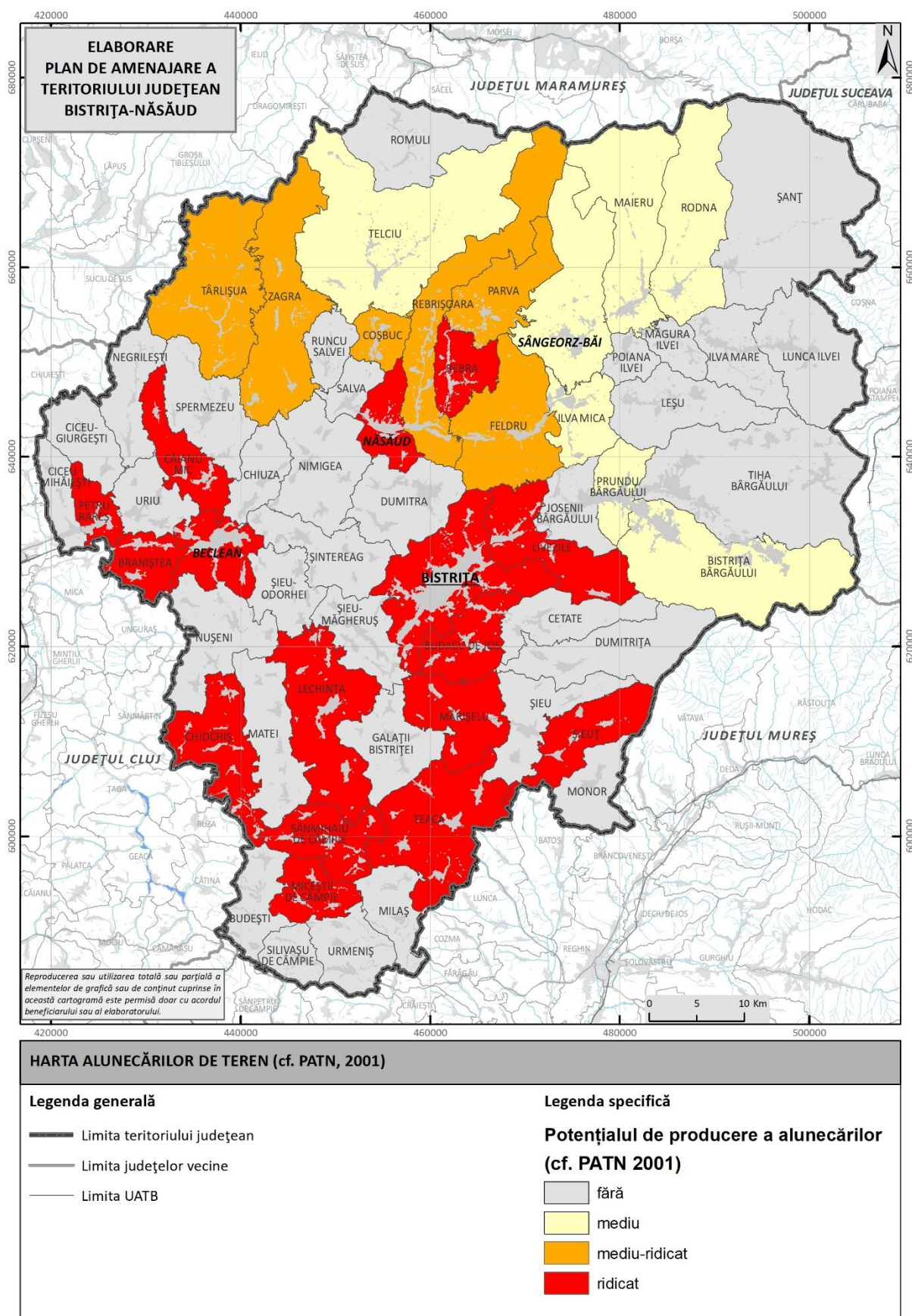
Fig. 2.25. ZONAREA UAT DUPĂ POTENȚIALUL DE PRODUCERE A ALUNECĂRIILOR DE TEREN CONFORM SECȚIUNII V, ZONE DE RISC NATURAL, 2001.
