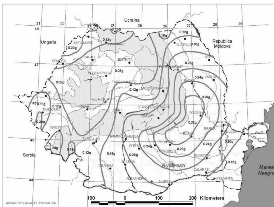
Fig. 2.51. ZONAREA TERITORIULUI ROMÂNIEI ÎN TERMENI DE VALORI DE VÂRF ALE ACCELAȚIEI TERENULUI PENTRU PROIECTARE AG PENTRU CUTREMURE AVÂND INTERVALUL MEDIU DE RECURENȚĂ IMR = 100 ANI
