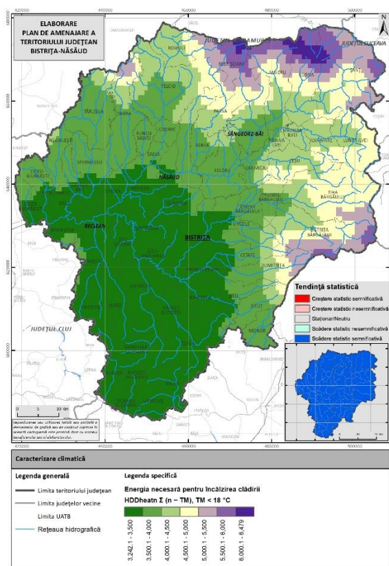
Fig. 2.62. ENERGIA NECESARĂ PENTRU ÎNCĂLZIREA CLĂDIRILOR (HDDHEATH)
