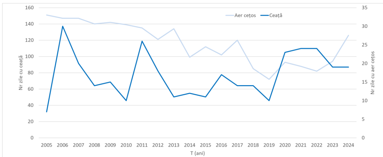
Fig. 2.68. ZILELE CU CEAȚĂ ȘI AER CEȚOS ÎNREGISTRATE LA STAȚIA BISTRIȚA
