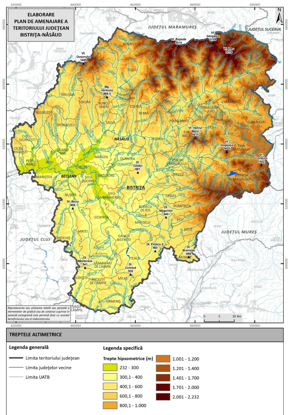
Fig. 2.4 HARTA HIPSOMETRICĂ
