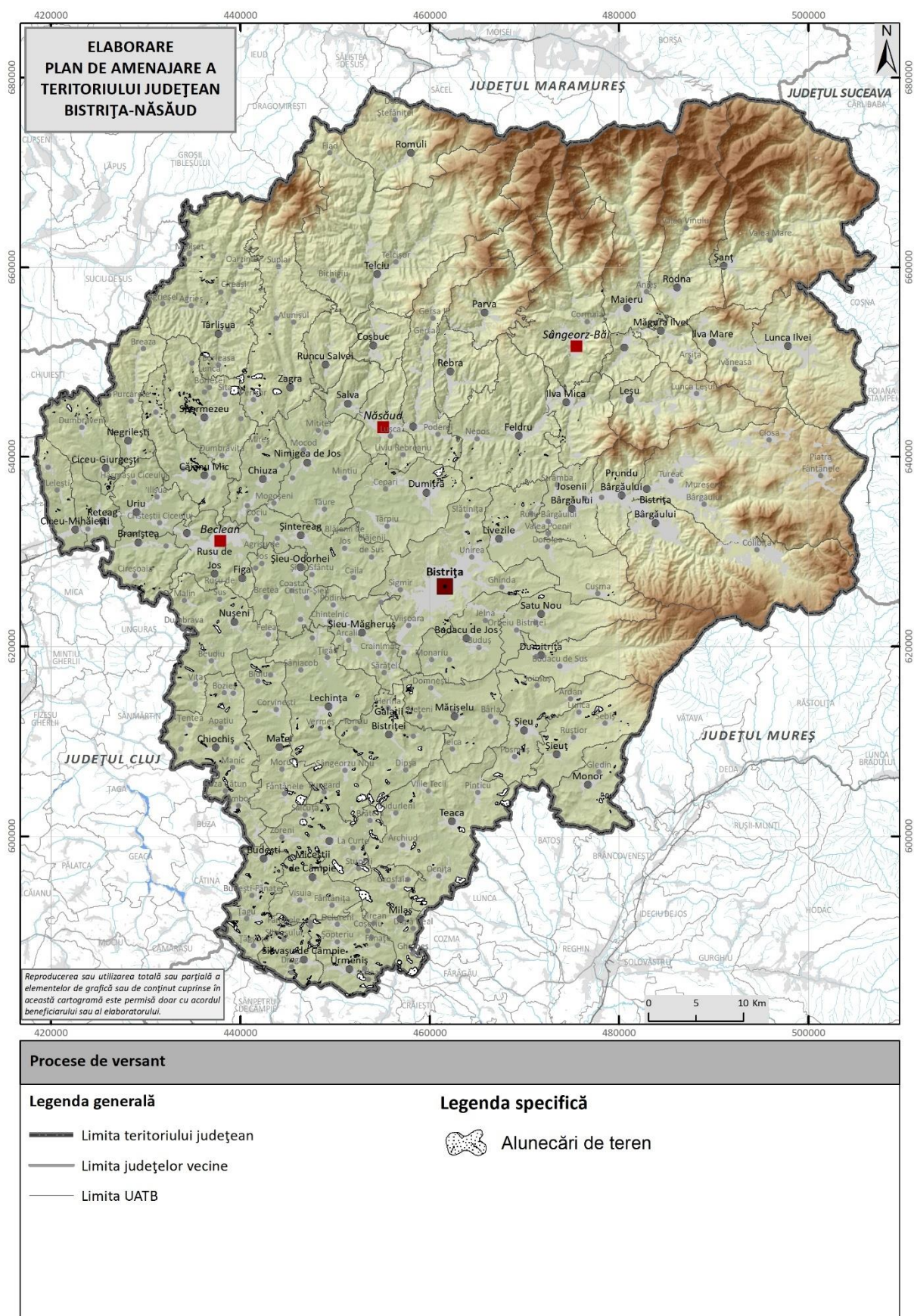
Fig. 2.26. DISTRIBUȚIA PROCESELOR DE VERSANT DIN JUDEȚUL BISTRIȚA NĂȘĂUD.
