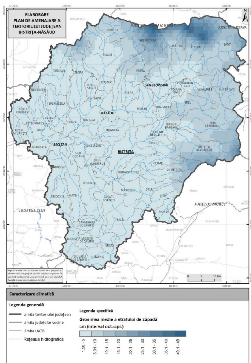
Fig. 2.25. GROSIMEA MEDIE A ZĂPEZII ÎN JUDEȚUL BISTRITĂ-NĂSĂUD PENTRU PERIOADA 2004-2024. Sursa: date prelucrate după baza de date furnizată de ANM
