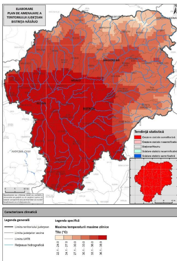
Fig. 2.53. MAXIMA TEMPERATURII MAXIME ZILNICE
