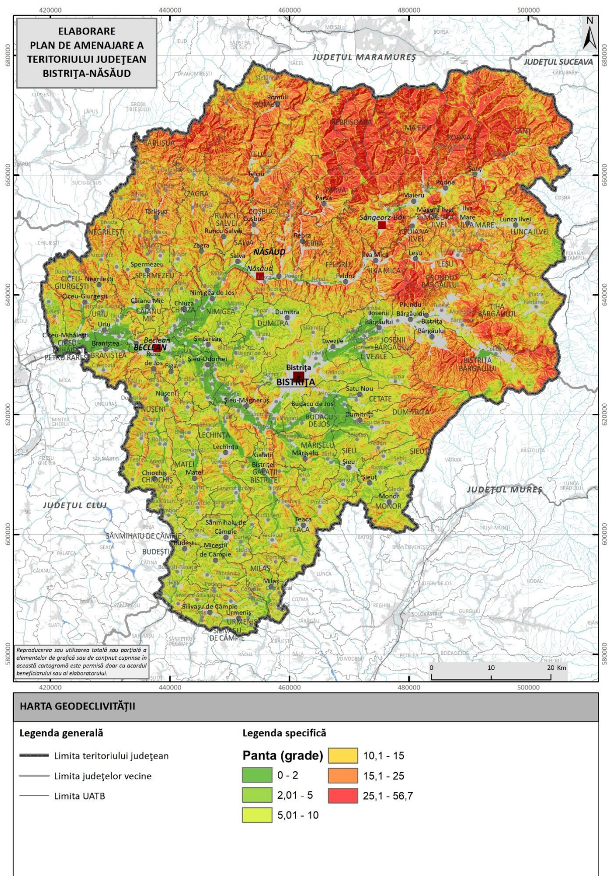
Fig. 2.28. HARTA PANTELOR DIN JUDEȚUL BISTRIȚA NĂȘĂUD
