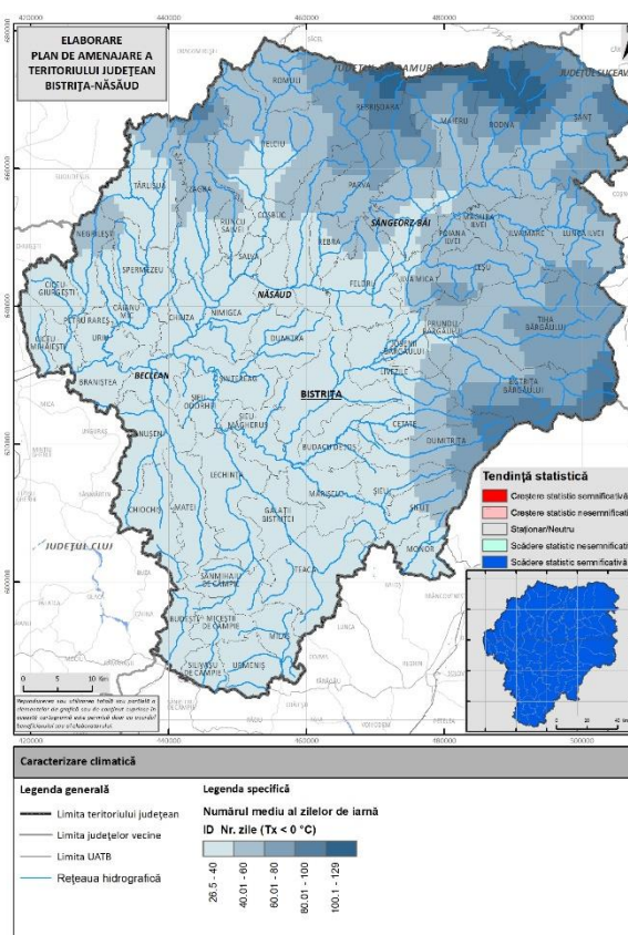
Fig. 2.56. ZILE DE IARNĂ
