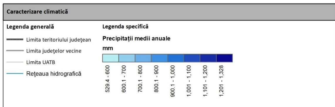
Fig. 2.20 CANTITĂȚI DE PRECIPITAȚII MEDII ANUALE ÎN JUDEȚUL BISTRIȚA-NĂȘAUD 1961-2024. Sursa: date prelucrate după baza de date furnizată de ANM
