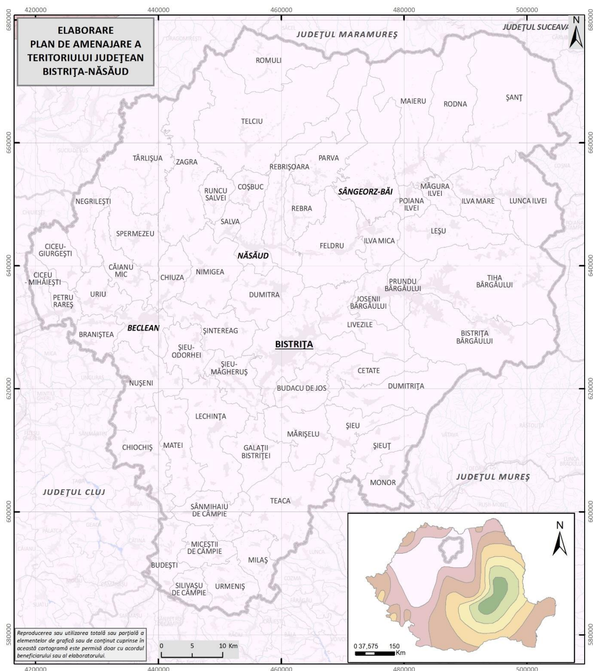
Harta zonării valorilor de vârf ale accelerației terenului pentru proiectare ag cu IMR = 225
