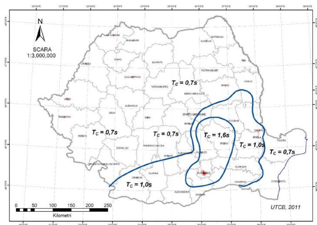
Fig. 2.23. HARTA ZONĂRII TERITORIULUI ÎN TERMENI DE PERIOADĂ DE COLȚ, T_c A SPECTRULUI DE RĂSPUNS (MDRAP, 2013).
