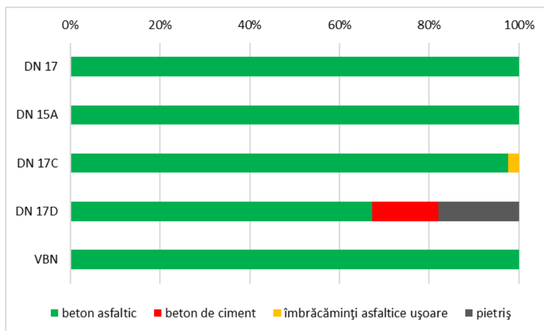
Fig. 2.3 STRUCTURA ÎMBRĂCĂMINȚII RUTIERE ȘI PONDEREA ACESTEIA DIN LUNGIMEA FIECĂRUI DRUM NAȚIONAL DIN JUDEȚUL BISTRIȚA-NĂSĂUD (2024)
