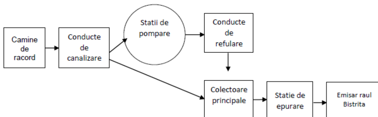
Fig. 2.30 CONFIGURATIE SISTEM DE CANALIZARE AGLOMERAREA BISTRIȚA
