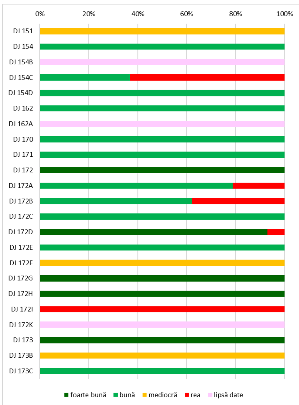
Fig. 2.9 STAREA DE VIABILITATE ȘI PONDERA ACESTEIA DIN LUNGIMEA FIECĂRUI DRUM JUDEȚEAN DIN JUDEȚUL BISTRIȚA-NĂSĂUD (2024)
