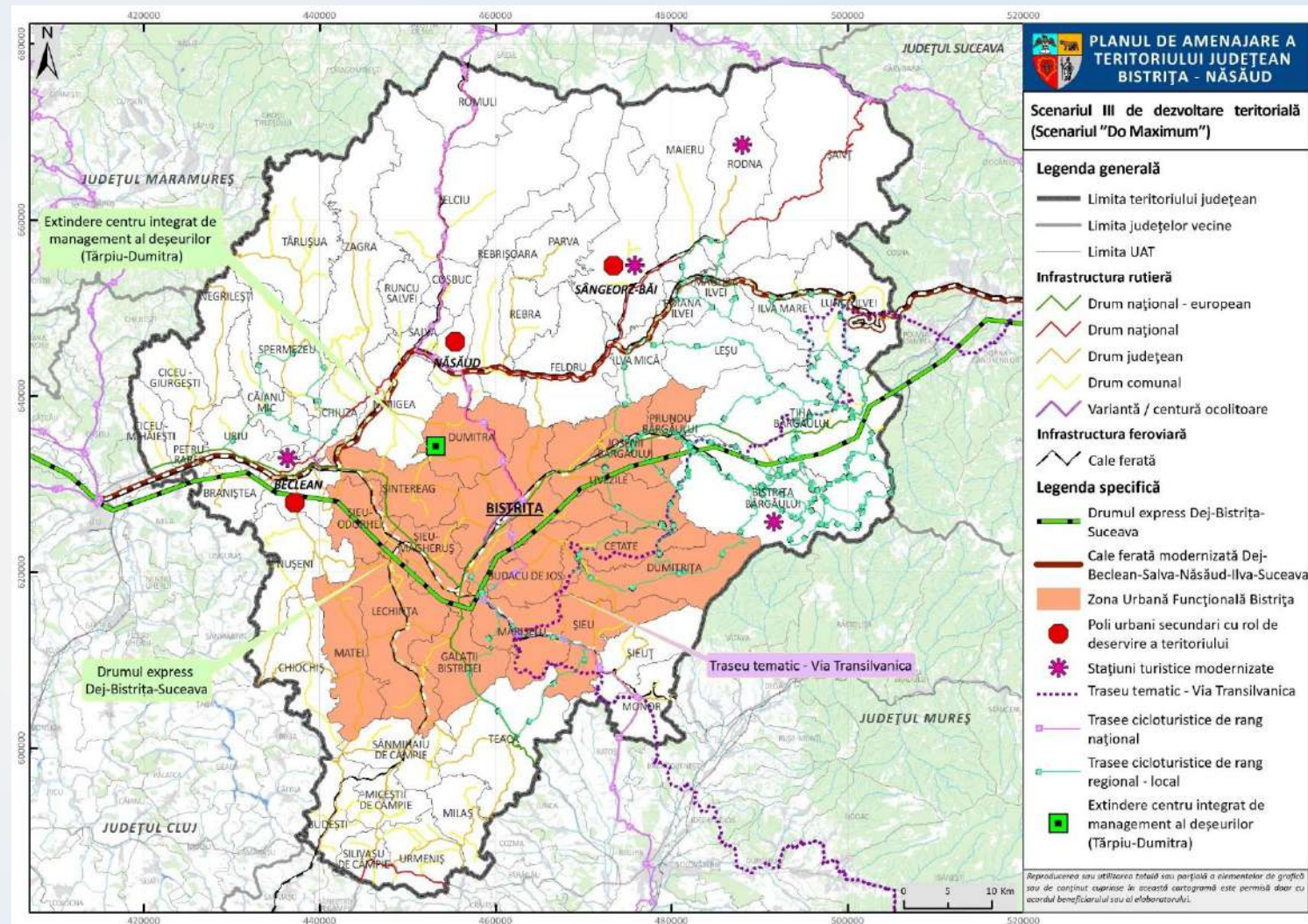
Scenariul III de dezvoltare teritorială (Scenariul "Do Maximum")
