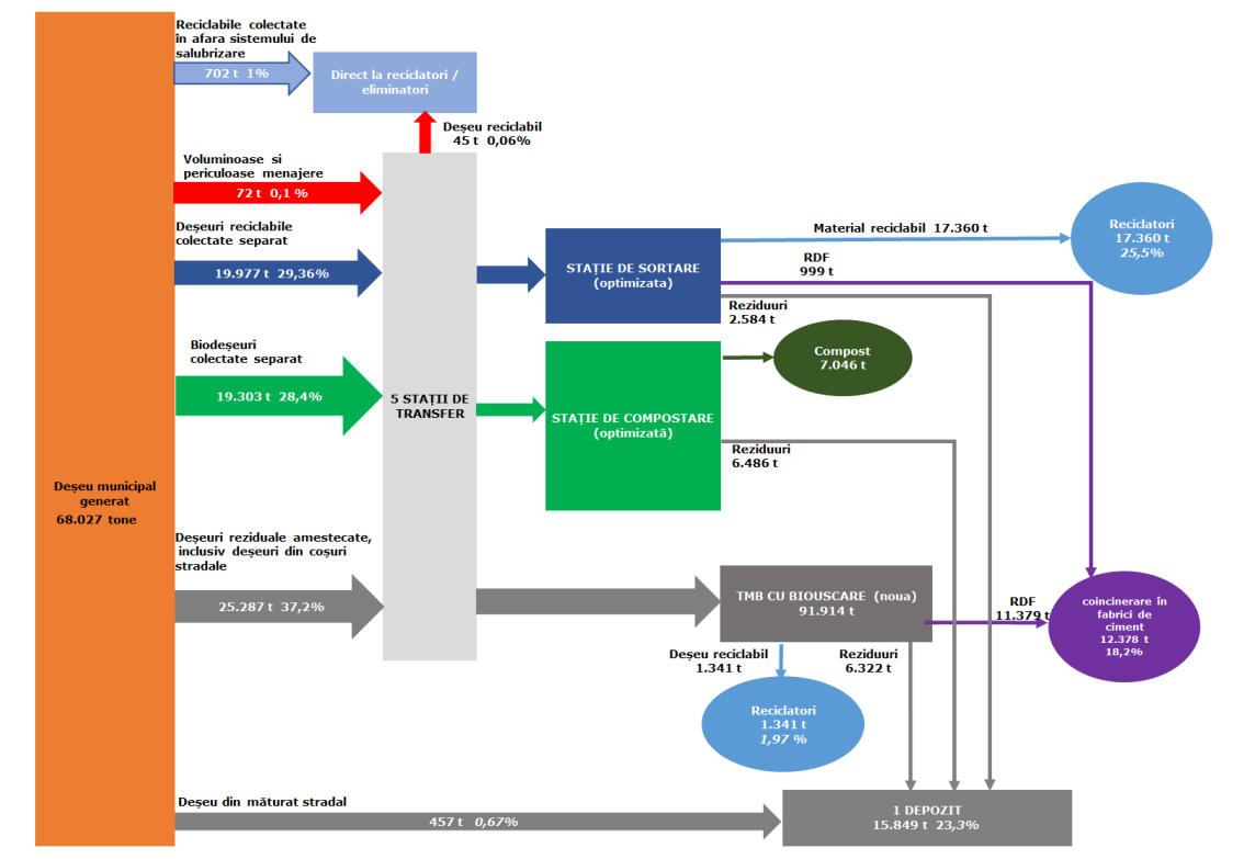
Figura 7-25 Schema fluxului tehnologic pentru Alternativa 1
