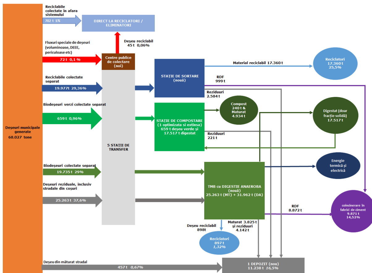
Sistemul de gestionare al deșeurilor municipale jud Bistrița-Nasaud, 2025, Alternativa 2
