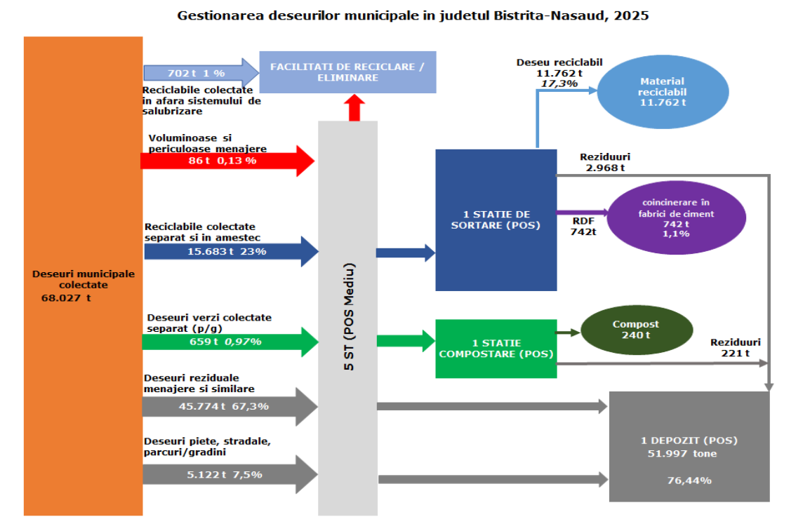
Figura 7-23 Schema fluxului tehnologic 2025, Alternativa „zero”
