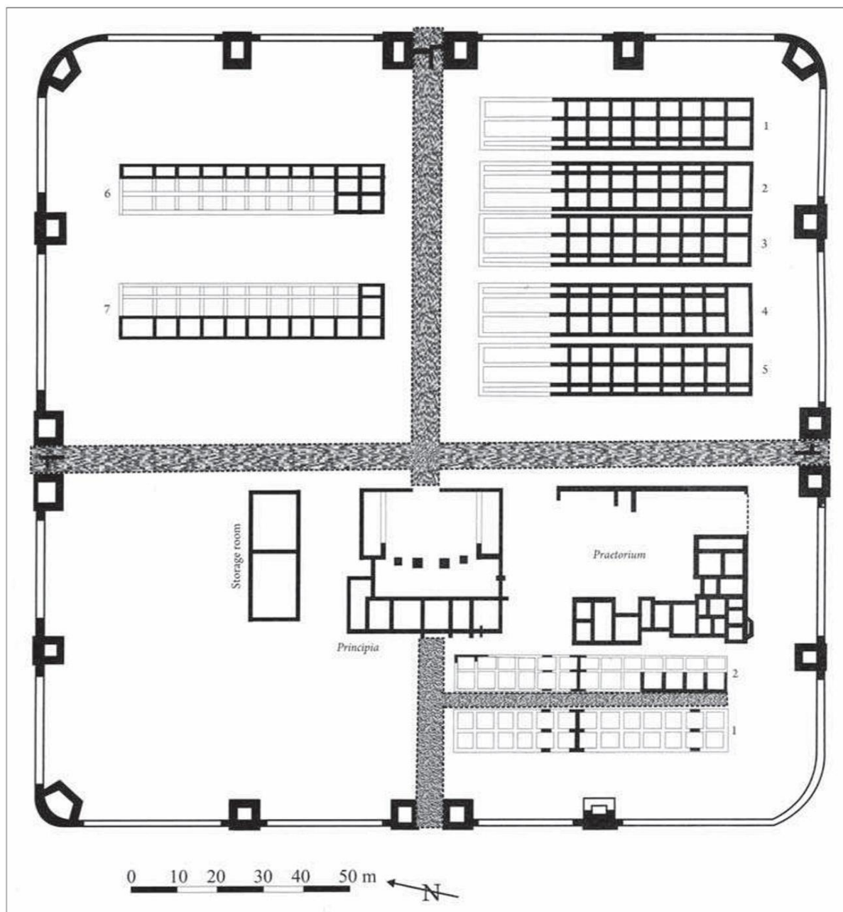
Fig. 3. Planul castrului auxiliar de la Ilișua.
