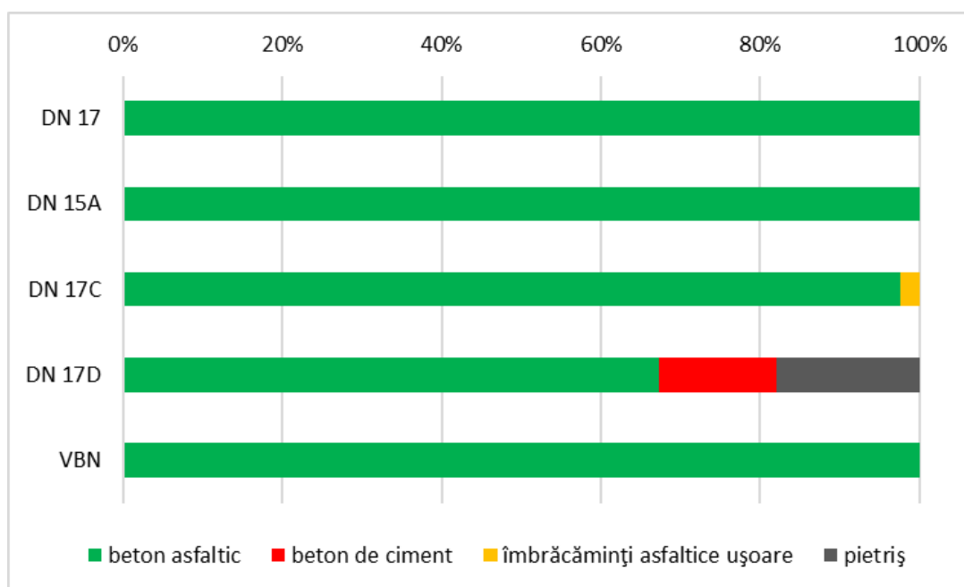
Fig. 2.3 STRUCTURA ÎMBRĂCĂMINȚII RUTIERE ȘI PONDERA ACESTEIA DIN LUNGIMEA FIECĂRUI DRUM NAȚIONAL DIN JUDEȚUL BISTRIȚA-NĂSĂUD (2024)
