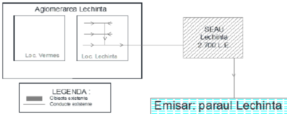
Fig. 2.34 SCHEMA SISTEMULUI DE CANALIZARE DIN AGLOMERAREA LECHINTA
