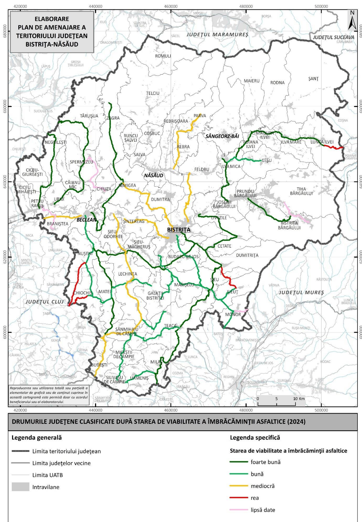
Fig. 2.10 DRUMURILE JUDEȚENE DIN JUDEȚUL BISTRIȚA-NĂȘĂUD CLASIFICATE DUPĂ STAREA DE VIABILITATE A ÎMBRĂCĂMINȚII ASFALTICE (2024)
