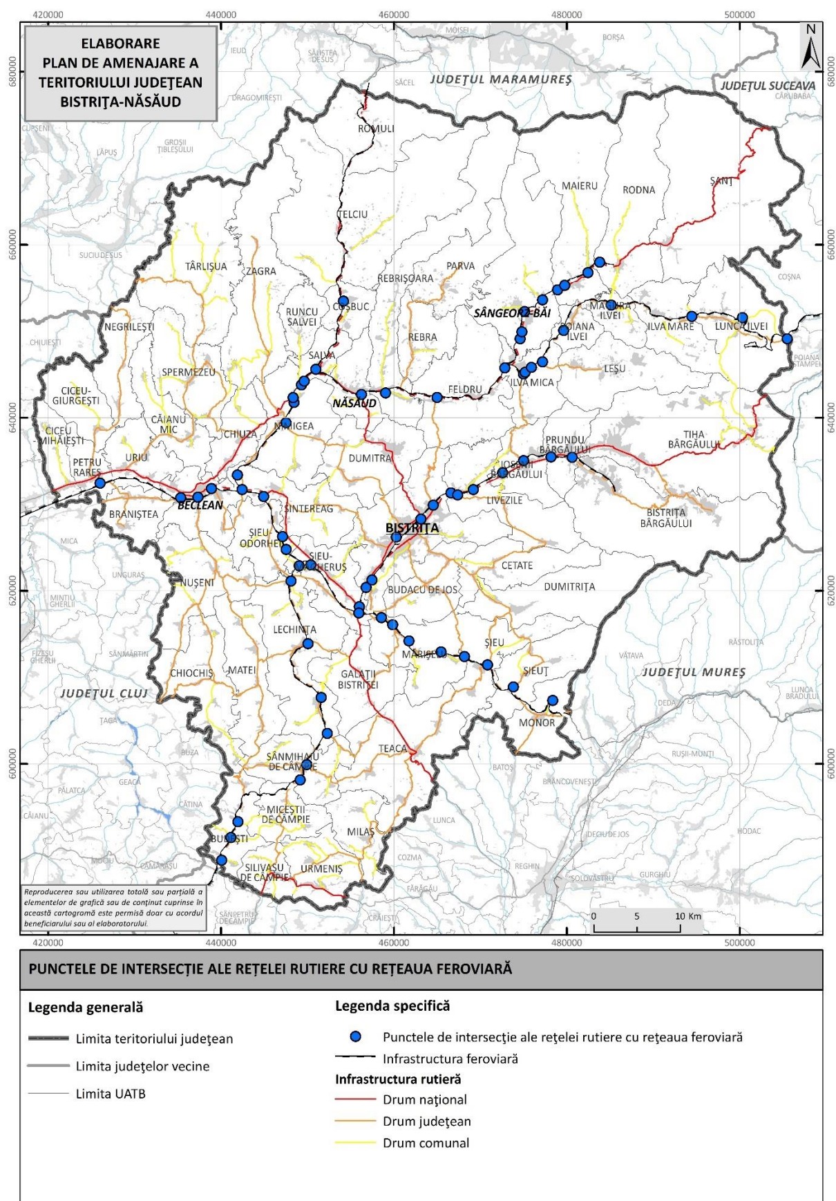
Fig. 2.12 PUNCTELE DE INTERSECȚIE ALE REȚELEI RUTIERE CU REȚEAUA FERROVIARĂ DIN JUDEȚUL BISTRITA-NĂSĂUD Sursa: autorii, 2025
