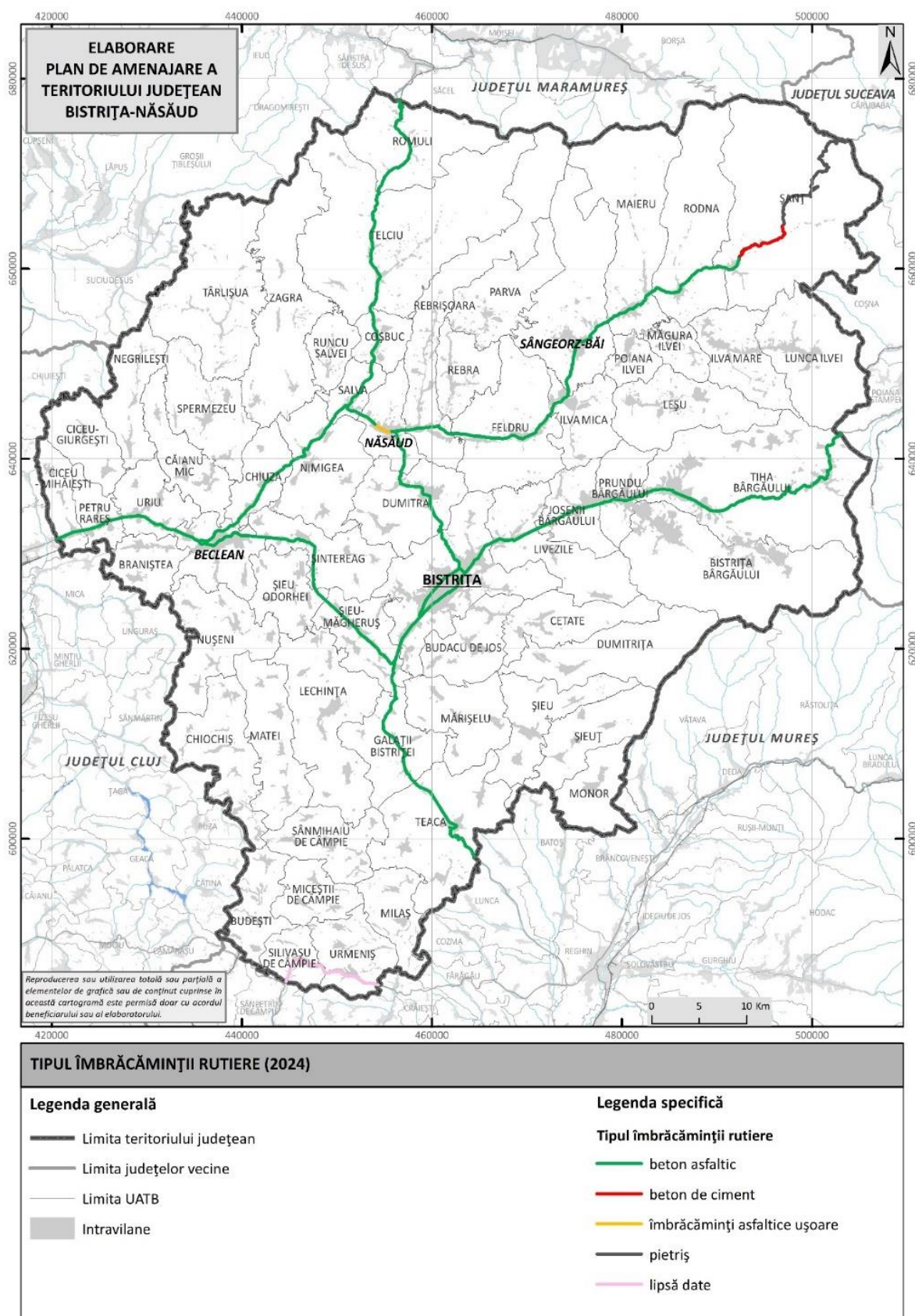
Fig. 2.4 DRUMURILE NAȚIONALE DIN JUDEȚUL BISTRIȚA-NĂȘĂUD CLASIFICATE DUPĂ TIPUL ÎMBRĂCĂMINȚII ASFALTICE (2024)
