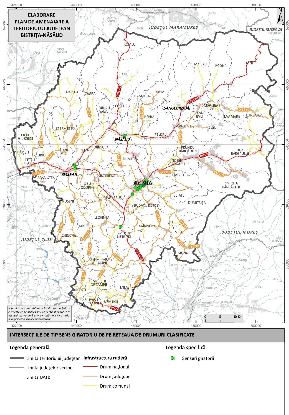
Fig. 2.11 INTERSECȚIILE DE TIP SENS GIRATORIU DE PE REȚEAUA DE DRUMURI CLASIFICATE DIN JUDEȚUL BISTRIȚA-NĂȘĂUD Sursa: autorii
