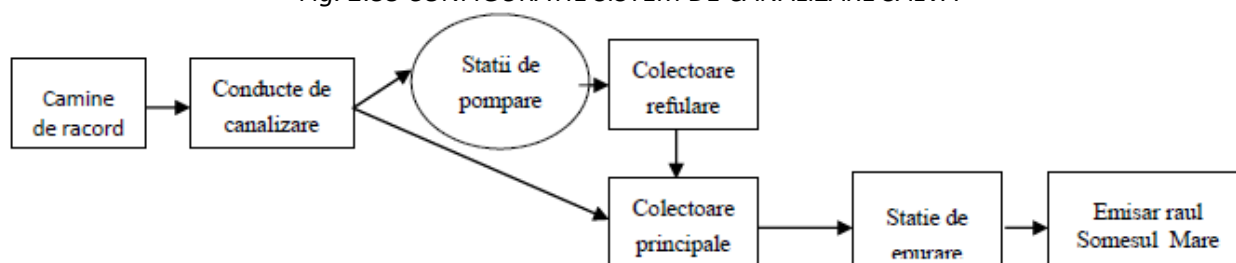
Fig. 2.33 CONFIGURATIE SISTEM DE CANALIZARE SALVA
