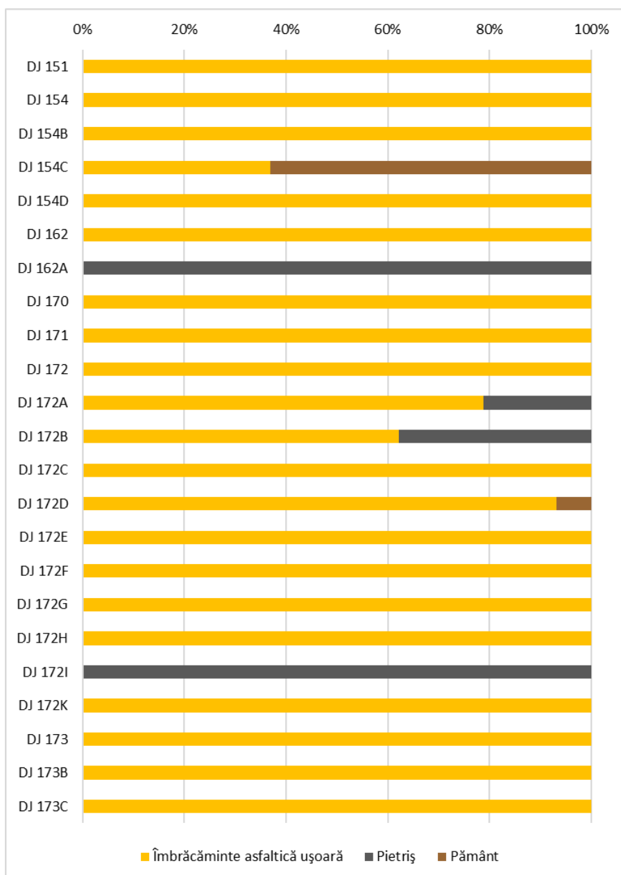
Fig. 2.5 STRUCTURA ÎMBRĂCĂMINȚII RUTIERE ȘI PONDEREA ACESTEIA DIN LUNGIMEA FIECĂRUI DRUM JUDEȚEAN DIN JUDEȚUL BISTRIȚA-NĂSĂUD (2024)
