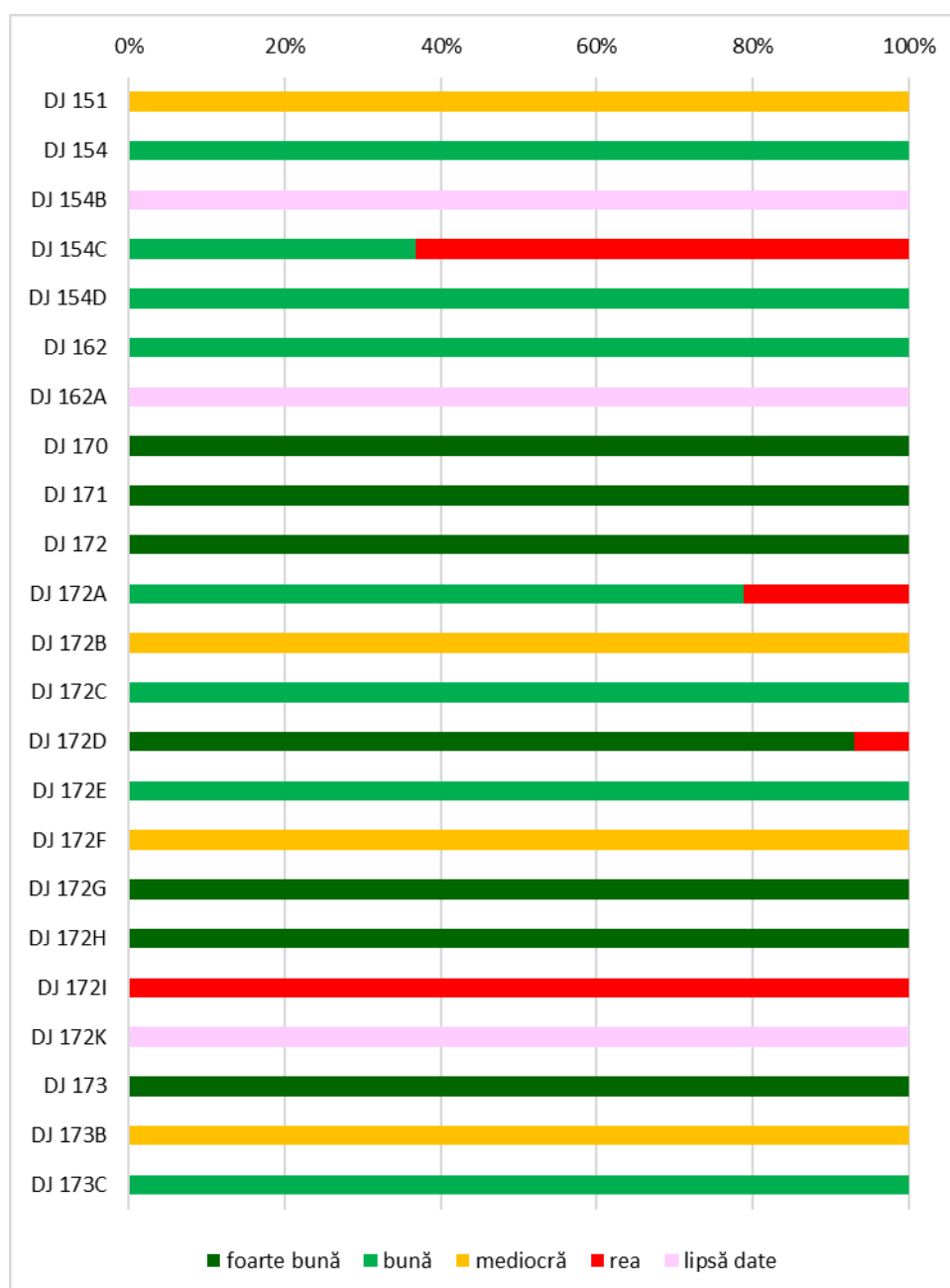
Fig. 2.9 STAREA DE VIABILITATE ȘI PONDERA ACESTEIA DIN LUNGIMEA FIECĂRUI DRUM JUDEȚEAN DIN JUDEȚUL BISTRIȚA-NĂSĂUD (2025)
